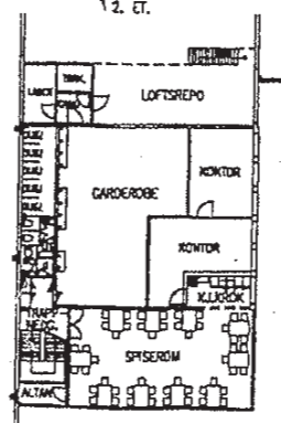
PLAN 2. ETG.
